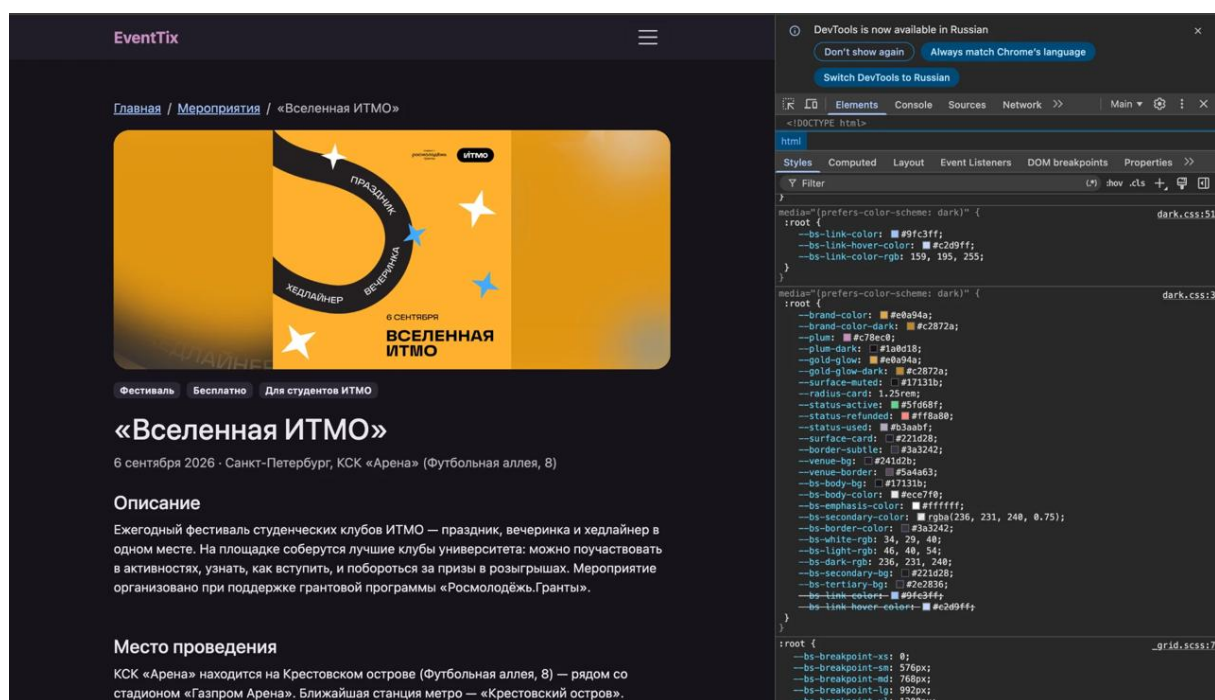
Рис. 4: DevTools: значения переменных берутся из файла тёмной темы, правила вёрстки — общие.
